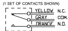
SPDT K24
