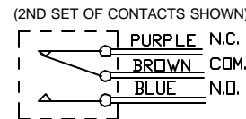
DPDT- P25
